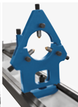
▲ Luneta fija cerrada (ROMI C470/C570/C670)
