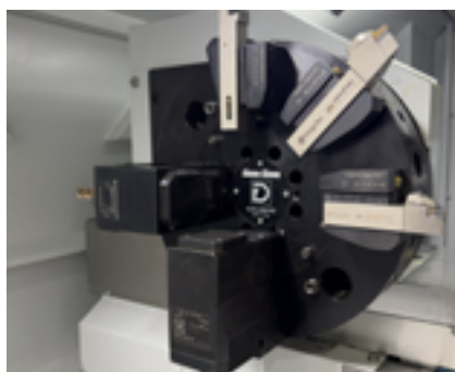
Torre eléctrica trasera de 8 posiciones de eje horizontal con herramientas accionadas VDI 30 (opcional) ▶
