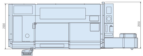
VISTA SUPERIOR
