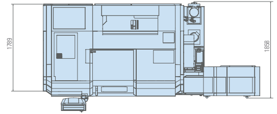
VISTA SUPERIOR
