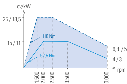
Cabezal 10.000 rpm
