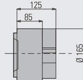
Placa hidráulica BH (*)
