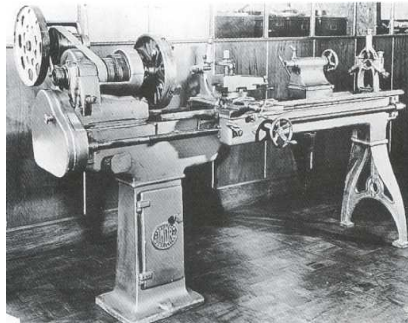
Torno mecânico modelo TP - 1941
